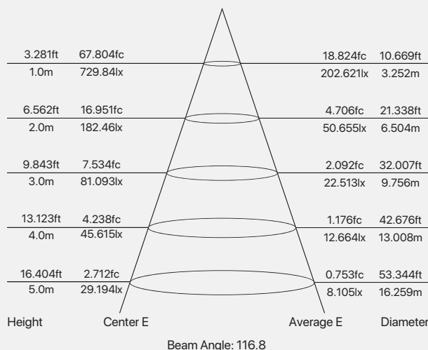
Curva de distribución luminosa
