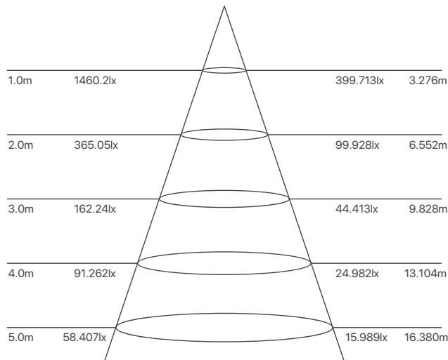
Curva de distribución luminosa
